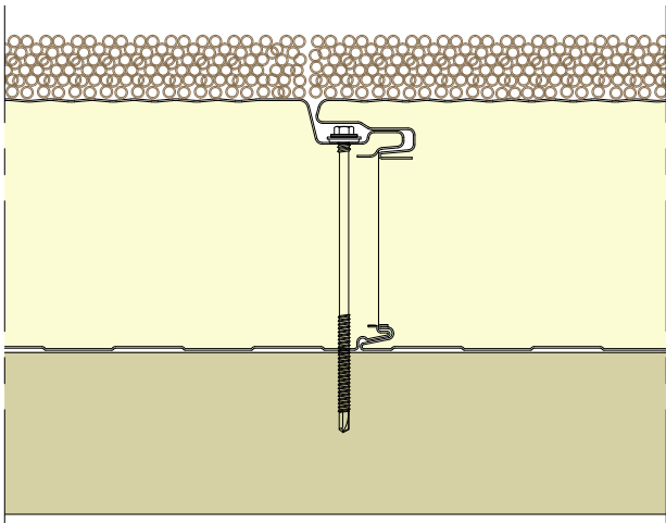
Schroefpositie (blind bevestigd)
